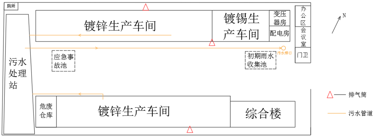
图 3-4 厂区平面布置图
