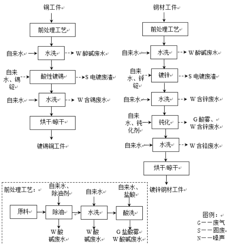
图 3-5 生产工艺流程及产污环节示意图
