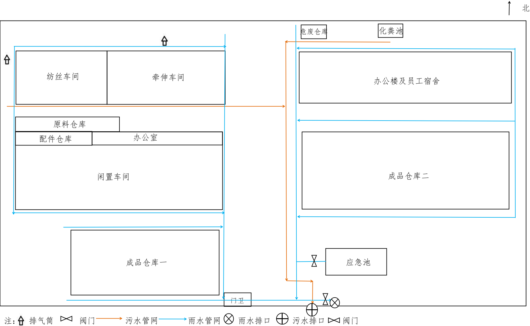
附件 6 企业雨、污水管网及重要阀门布置图
