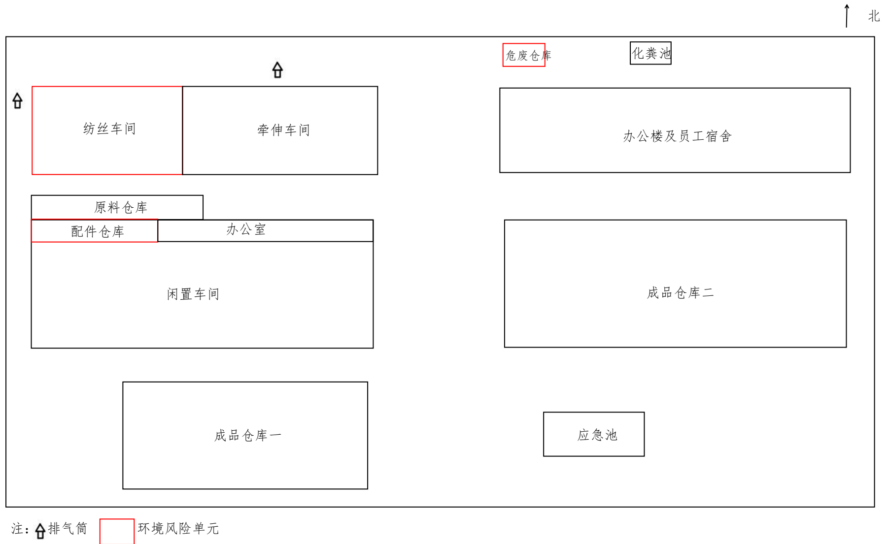
附件 10 企业风险源及监控点平面图
