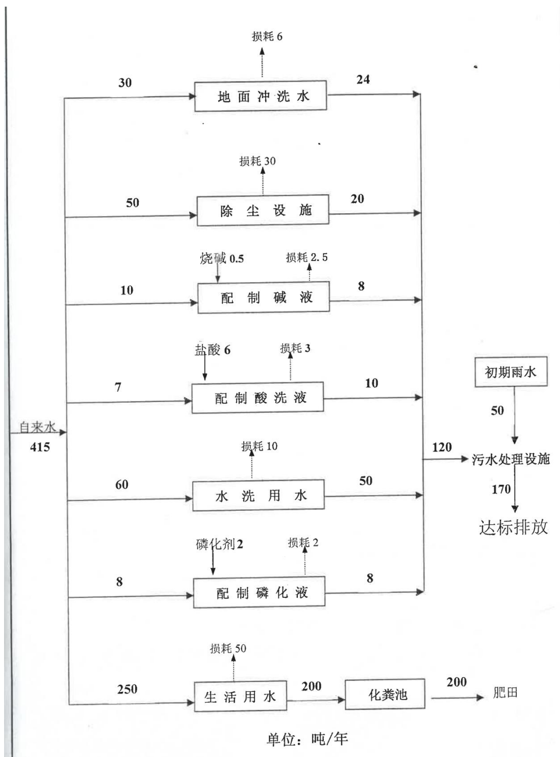
图 3 验收时水平衡图
