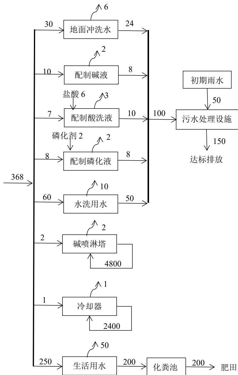
图 4 变动后水平衡图（单位：吨/年）
