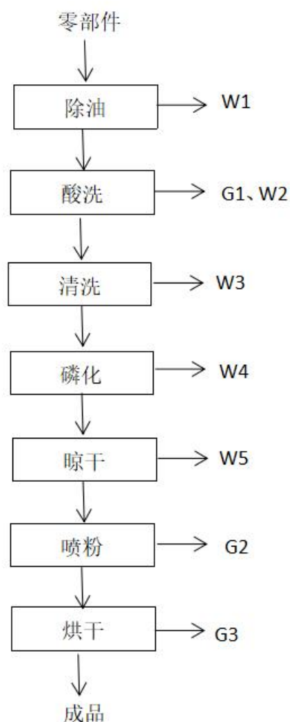
图3 验收生产工艺流程图
