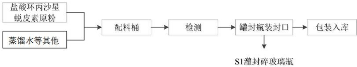
图4-1 蚕用口服液 (克菌灵液、蜕皮素)生产工艺流程及产污节点图
