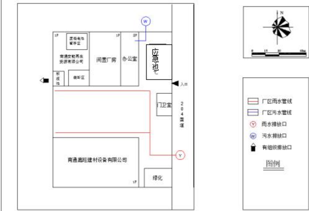
图4-4 场地总平面布置图
