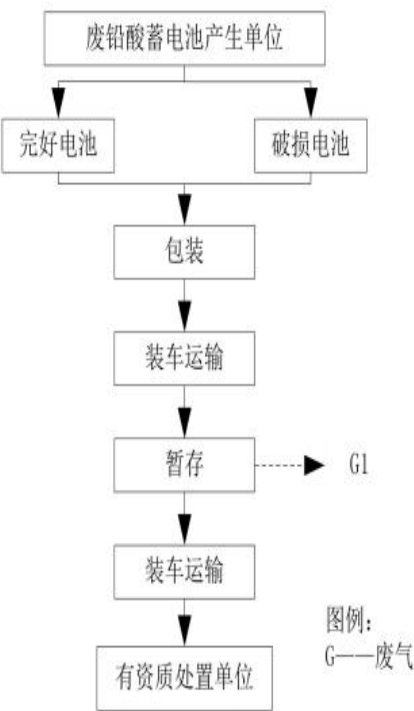
图4-1 生产工艺流程及产污节点图
