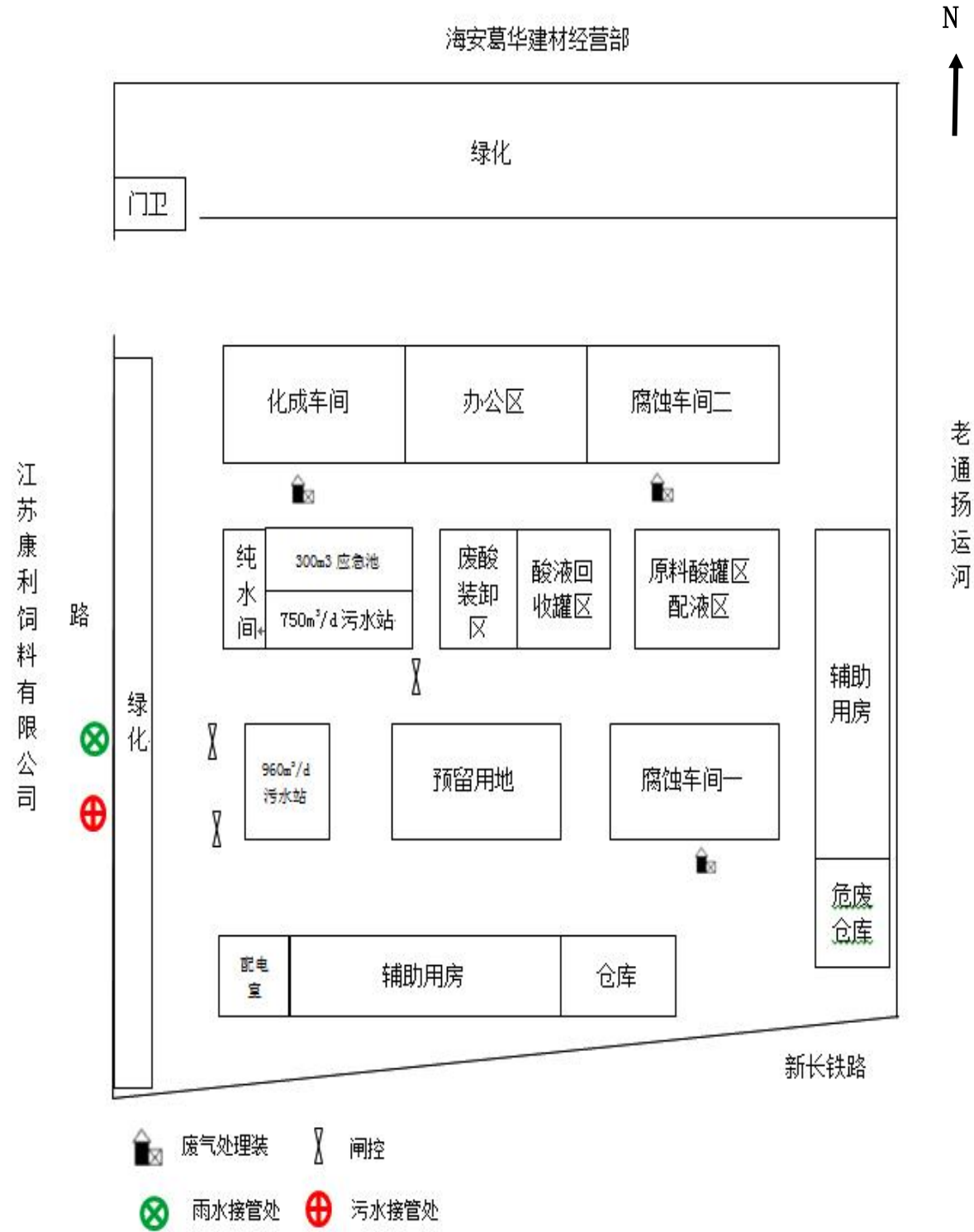
附图 B3 项目厂区平面布置图
