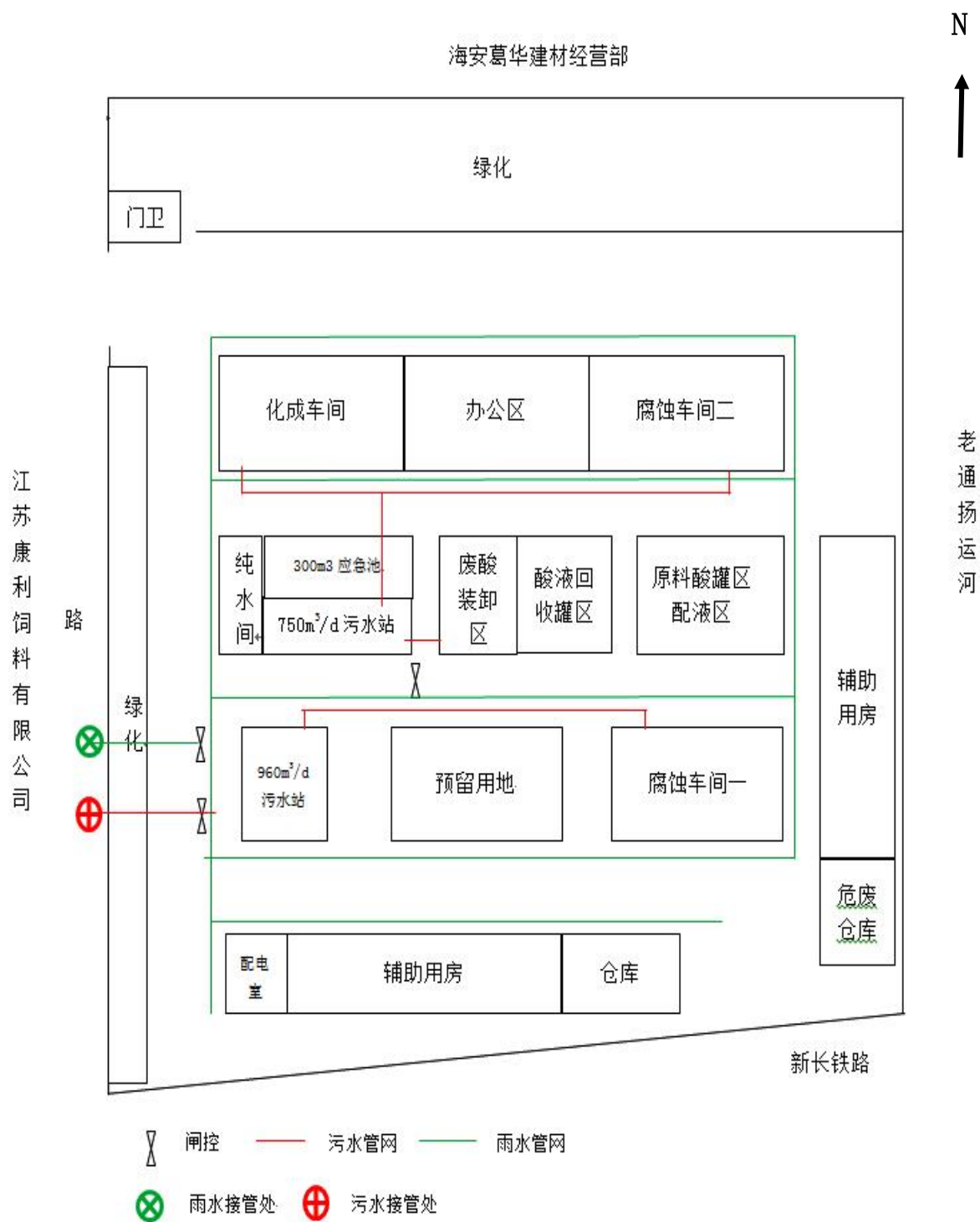
附图 B6 项目雨污管网分布图
