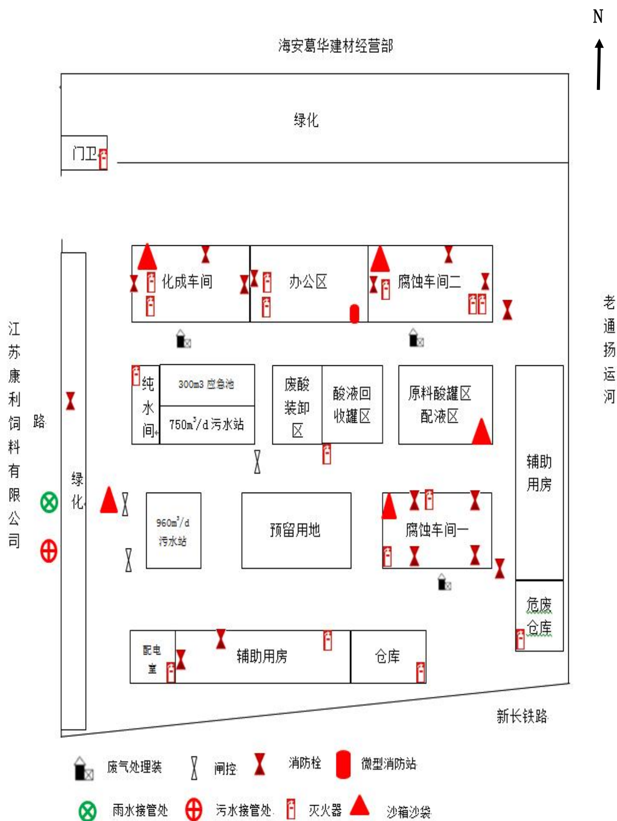
附图 B7 项目消防器材、应急物资布置图
