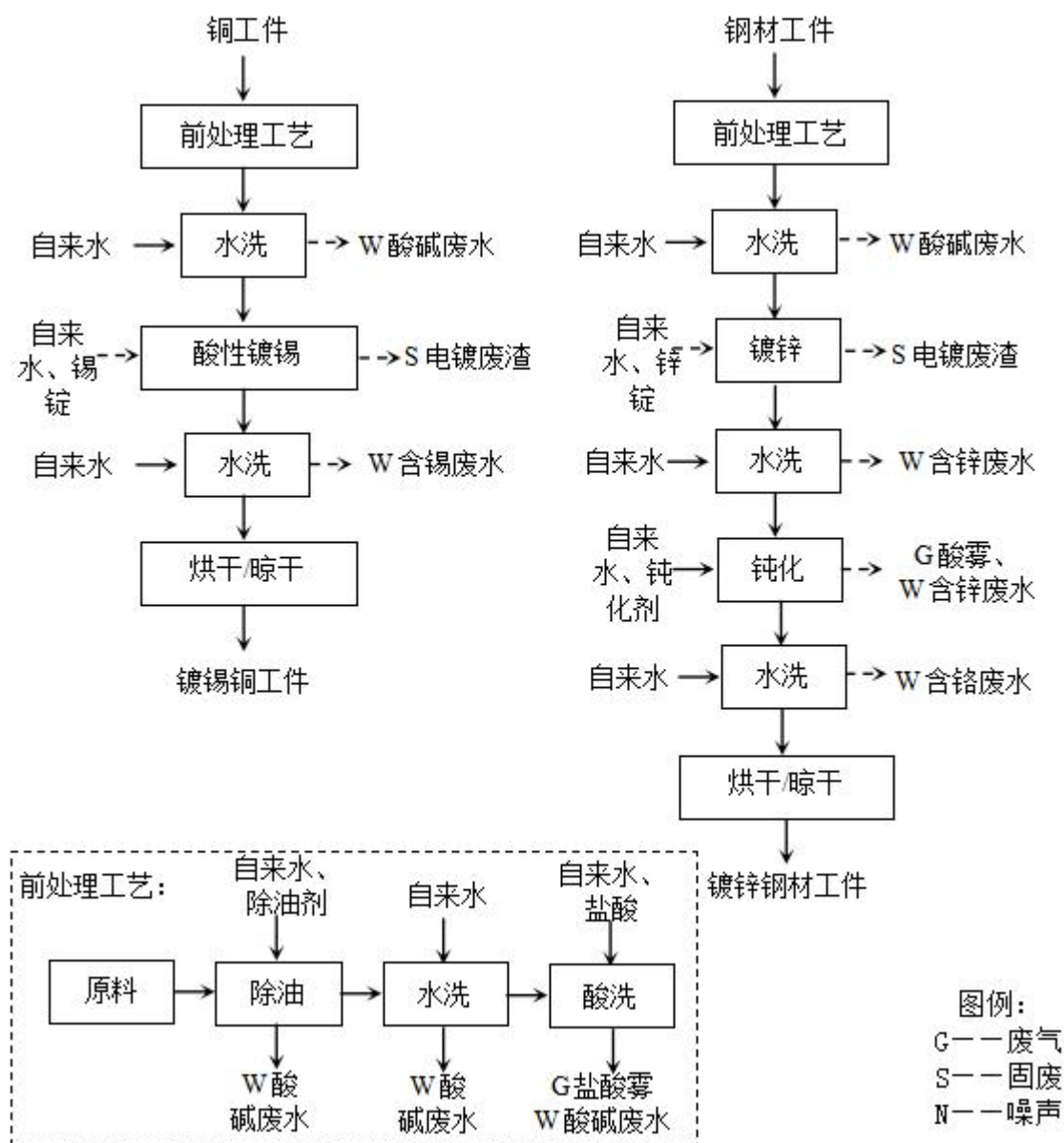
图4-1 生产工艺流程及产污节点图
